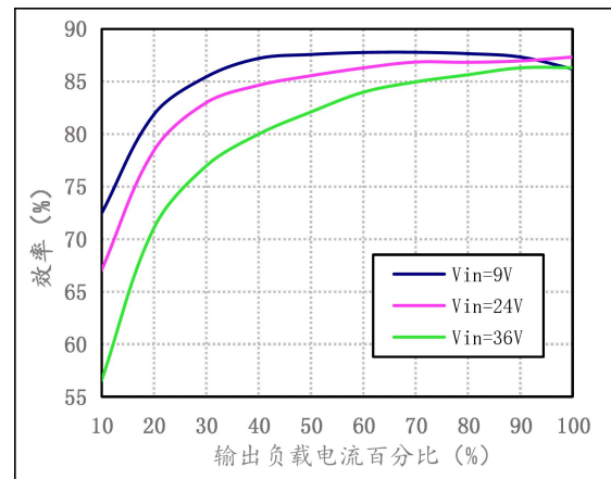
效率曲线 ( V_o=12V )
