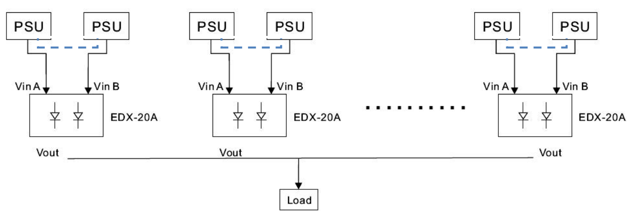
3.4 可靠性系统构建图 Reliability system:
