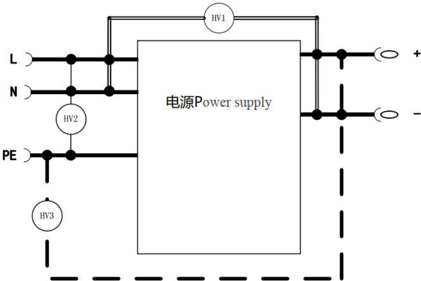
高压测试high-voltage test
