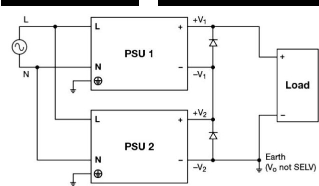
3.2 1+1 冗余接线图 1+1 Redundancy Connection Diagram
