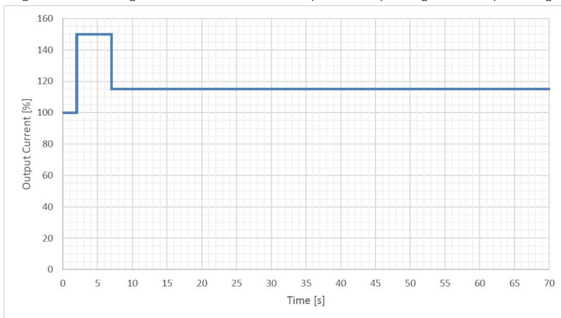
图2: 短路情况下，非重复的峰值电流特性
