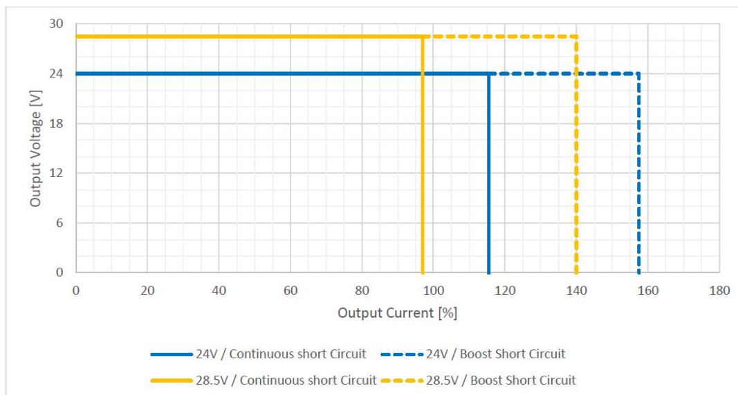
图1: 不同输出电压下，正常和峰值工作时的限流曲线
