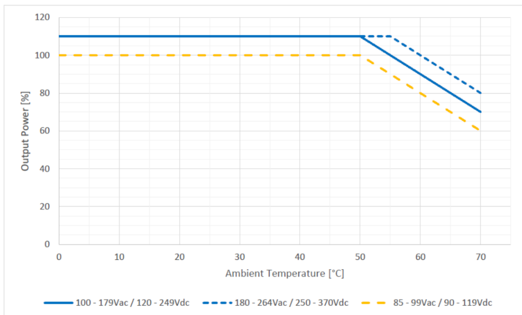
图2：环境温度和输入电压下输出功率降额曲线
